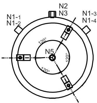
Alulnézet
