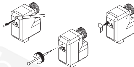
8. ábra S2 segédkapcsoló beállítása
