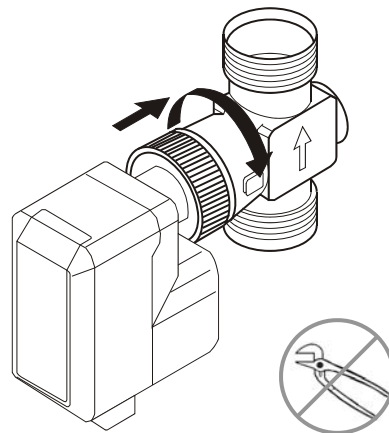
3. ábra Motor felszerelése
