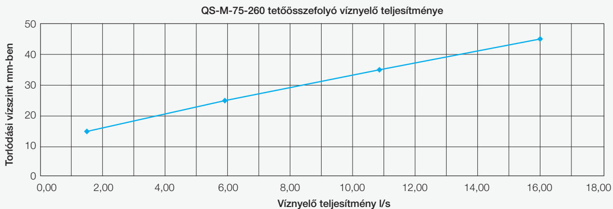
46. ábra: QS-M-75-260 tetőösszefolyó víznyelési teljesítmény grafikonja (DIN EN 1253)
